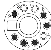
CEBORA® 6 pins
